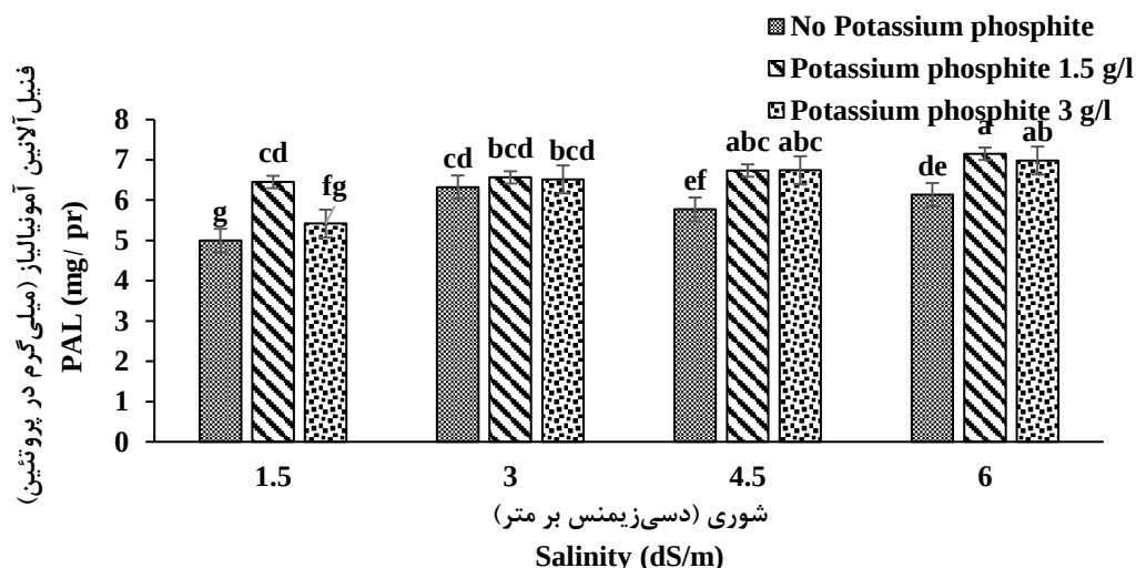
شکل ۳- برهمکنش تنش شوری و فسفیت پتاسیم بر فعالیت آنزیم فیل آلانین آمونیالیز در لیموترش. مقادیر، میانگین سه تکرار و حروف یکسان بیانگر عدم اختلاف معنی‌دار با آزمون توکی ( P < 0.05 ) است.
