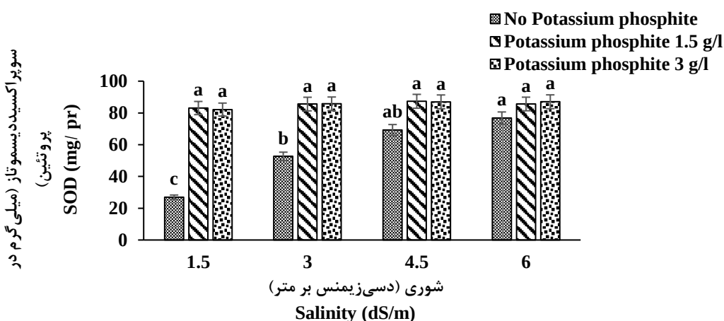
شکل ۴- برهمکنش تنش شوری و فسفیت پتاسیم بر فعالیت آنزیم سوپراکسید دیسموتاز در لیموترش. مقادیر، میانگین سه تکرار و حروف یکسان بیانگر عدم اختلاف معنی‌دار با آزمون توکی ( P < 0.05 ) است.
