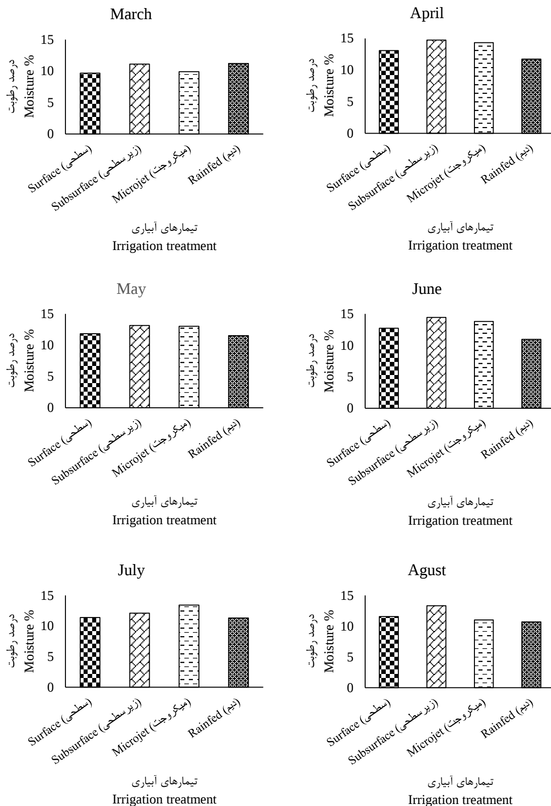
Fig. 2. Changes of mean moisture percentage in 60-90 cm soil depth for different supplemental irrigation methods. شکل ۲- تغییرات متوسط درصد رطوبت در عمق ۶۰-۹۰ سانتی متری خاک در روش‌های مختلف آبیاری تکمیلی.
