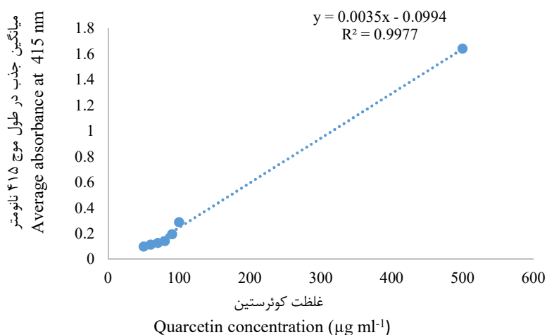
Fig. 2. Flavonoid standard (quarceetin) curve.
