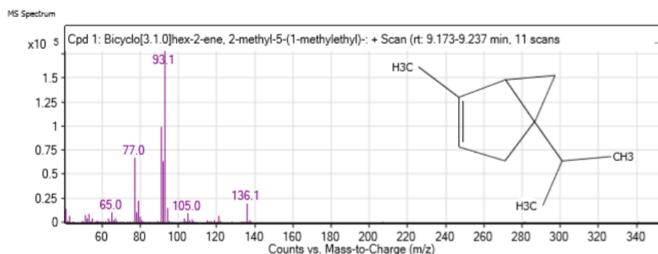
شکل ۱- نمونه نتایج تجزیه اسانس میخک هندی ( Syzygium aromaticum ) به روش GC/MS.
