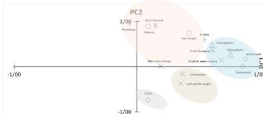
شکل ۱۵- بای پلات نژادگان‌های گواوا مورد بررسی بر اساس مولفه اول و دوم.
