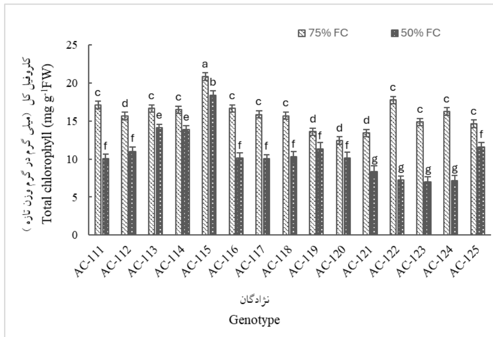
شکل ۳- برهمکنش رژیم آبیاری و نژادگان بر محتوای کلروفیل کل نژادگان‌های گواوا. مقادیر، میانگین سه تکرار و حروف یکسان بیانگر عدم اختلاف معنی‌دار با آزمون LSD ( P \leq 0.01 ) است.
