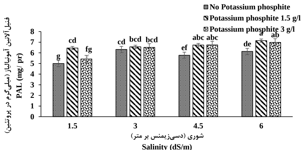
شکل ۳- برهمکنش تنش شوری و فسفیت پتاسیم بر فعالیت آنزیم فیل آلانین آمونیالایز در لیموترش. مقادیر، میانگین سه تکرار و حروف یکسان بیانگر عدم اختلاف معنی‌دار با آزمون توکی ( P < 0.05 ) است.
