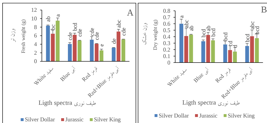
شکل ۴- برهمکنش طیف‌های مختلف نوری و رقم بر وزن تر و خشک گیاهچه‌های کشت بافتی سه رقم بگونیا رکس. Fig. 4. The interaction effect of different light spectra and cultivar on A) fresh and B) dry weight of tissue culture plantlets of three cultivars of Begonia rex .
