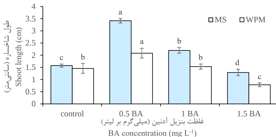
شکل ۷- اثر غلظت‌های مختلف BA و نوع محیط کشت بر طول شاخساره (سانتی‌متر). Fig. 7. The effect of different BA concentration and type of culture medium on shoot length (cm) parameter.
